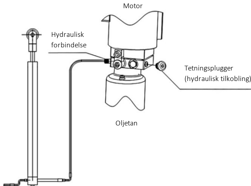
Figur: Tetningsplugg
