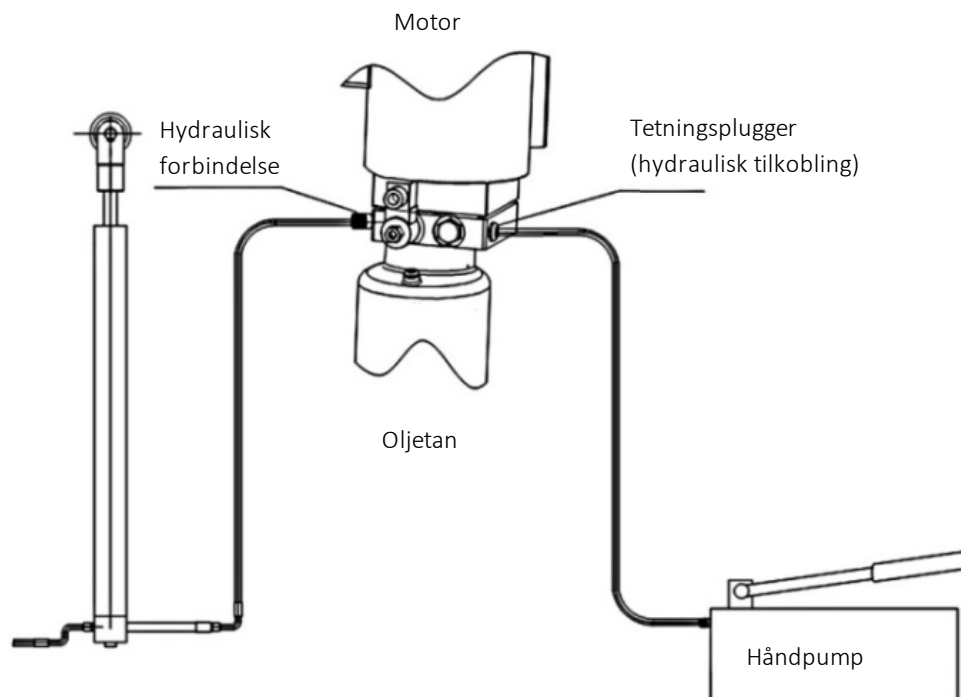
Figur: Håndpumpetilkoblinger
