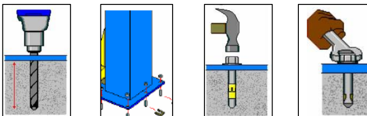
Figur: Arbeidstrinn for å feste søylene
