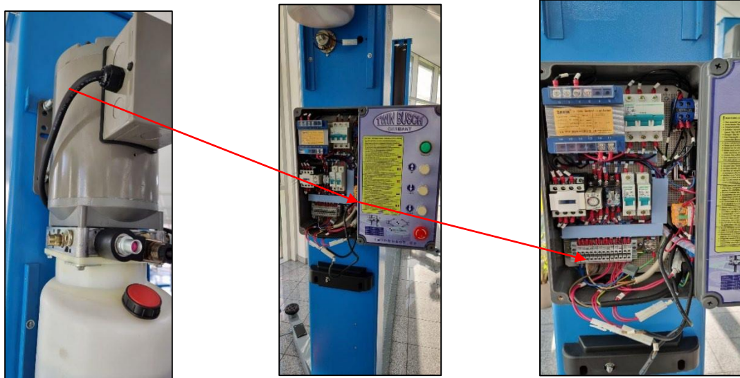
Figur: Koble strømforsyningen til kontrollenheten
