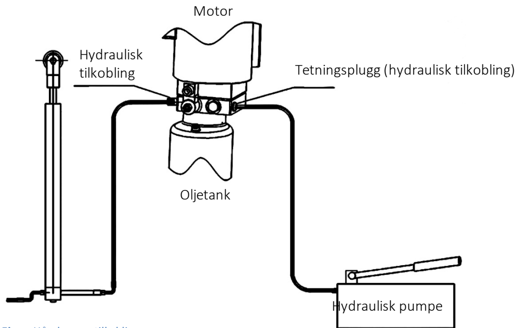
Figur: Håndpumpetilkoblinger
